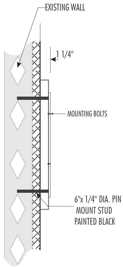
SECTION VIEW A-A N.T.S.
